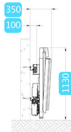
Plataforma plegada con fijación a pared
