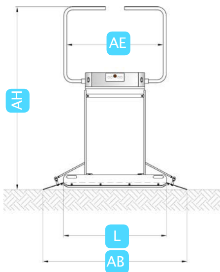
Plataforma totalmente abierta (embarque/desembarque en la planta baja)
